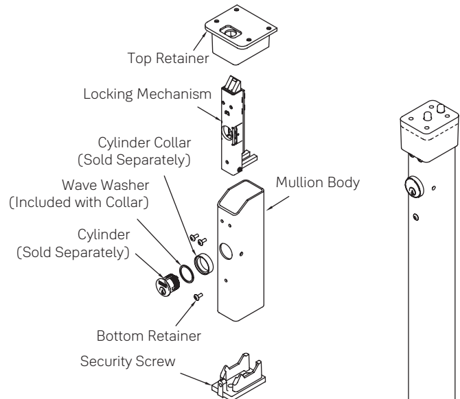
KRM200(F)
